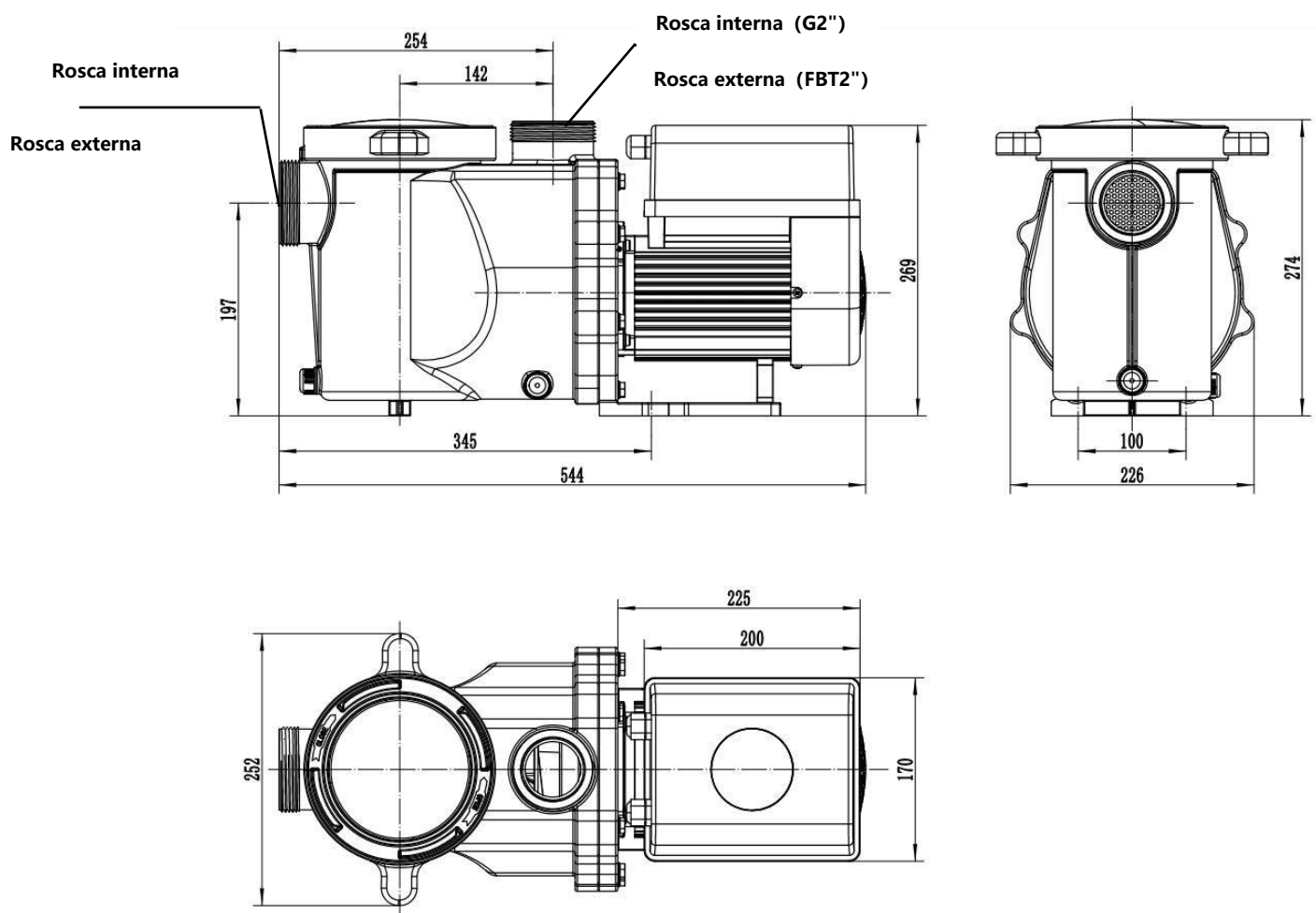
Figura 1 - Dimensión de la bomba
