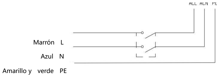
Figura 5 - Conector de entrada digital
